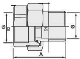
VTr.341 Сгон разъемный В-Н (американка)
