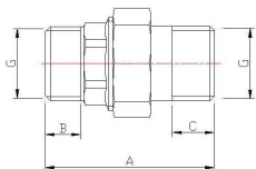
VTr.728 Сгон разъемный Н-Н (американка)
