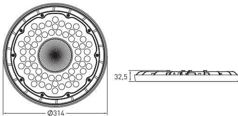
Рис. 3 - Габаритные размеры светильников ДСП-1103
