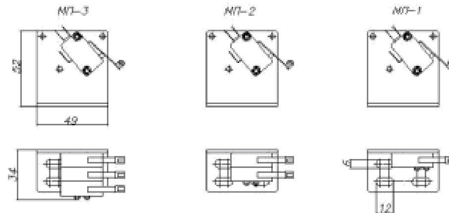
Блок-контакт для выключателей
