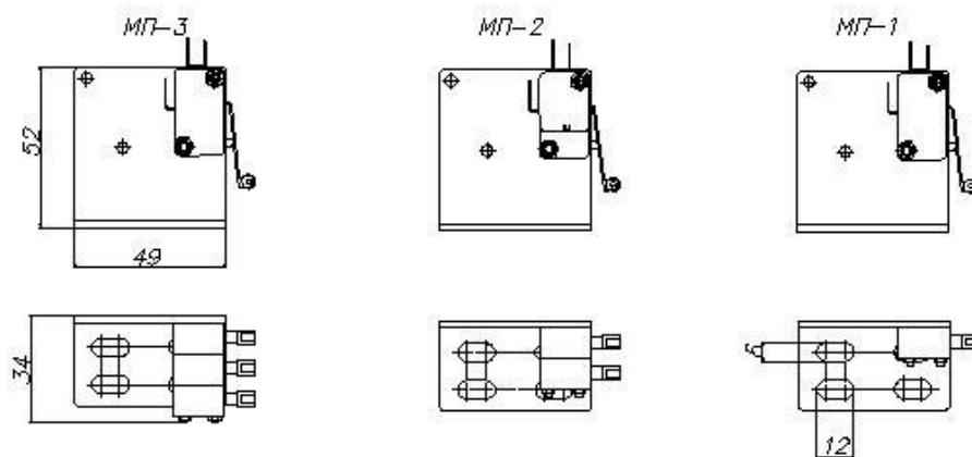
Блок-контакт для разъединителей
