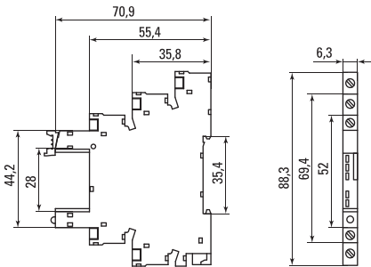
Рис. 3 Габаритные размеры PM Slim 23/1 EKF AVERES
