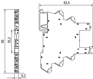
Рис. 4 Габаритные размеры PM slim 23/1 Push-in EKF AVERES
