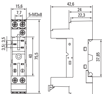
Рис. 1 Габаритные размеры PM Slim 25/1 EKF AVERES
