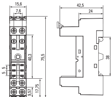
Рис. 2 Габаритные размеры PM Slim 22/2 EKF AVERES
