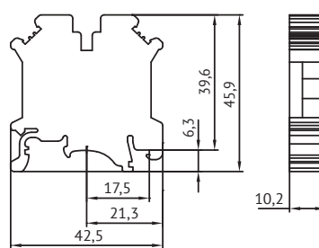
249859 Клемма проходная OptiClip TB-10-I-57A-(1,5-16)-серый 249860 Клемма проходная OptiClip TB-10-I-BU-57A-(1,5-16)-синий
