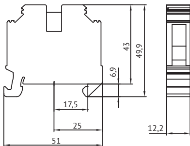
249861 Клемма проходная OptiClip TB-16-I-76A-(6-16)-серый 249862 Клемма проходная OptiClip TB-16-I-BU-76A-(6-16)-синий
