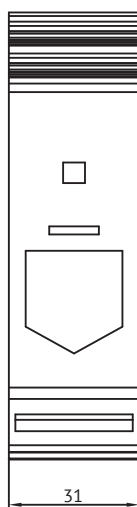
249871 Клемма проходная OptiClip ТВ-150-I-309A-(35-150)-серый
