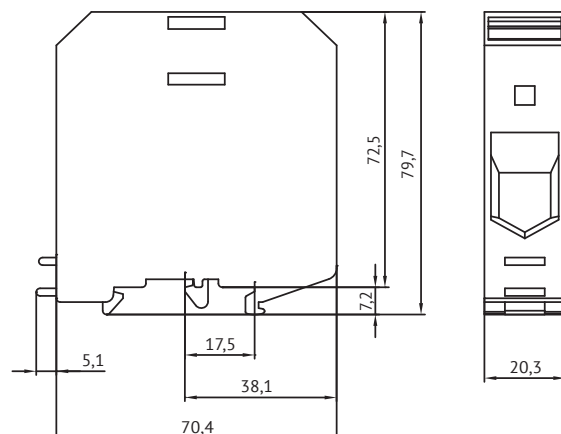
249867 Клемма проходная OptiClip TB-70-I-192A-(16-95)-серый 249868 Клемма проходная OptiClip TB-70-I-BU-192A-(16-95)-синий
