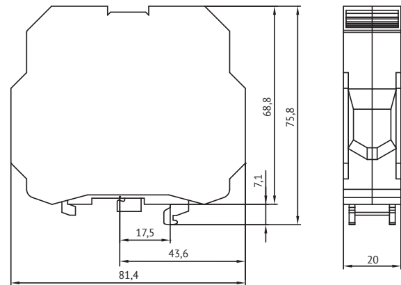
249881 Клемма заземляющая OptiClip ТВ-50-PE-I-150A-(16-50)-PEN
