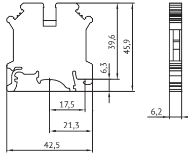
249859 Клемма проходная OptiClip TB-10-I-57A-(1,5-16)-серый 249860 Клемма проходная OptiClip TB-10-I-BU-57A-(1,5-16)-синий
