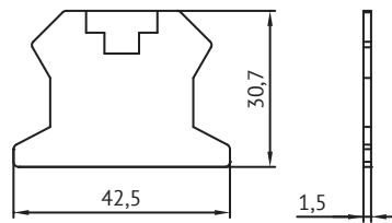
249891 Крышка концевая для клеммы проходной OptiClip D-TB-2,5-серый
