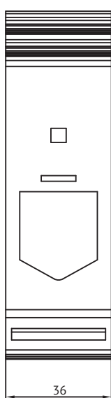
249873 Клемма проходная OptiClip ТВ-240-I-415A-(70-240)-серый
