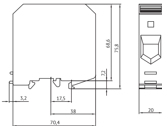
249865 Клемма проходная OptiClip TB-50-I-150A-(16-70)-серый 249866 Клемма проходная OptiClip TB-50-I-BU-150A-(16-70)-синий
