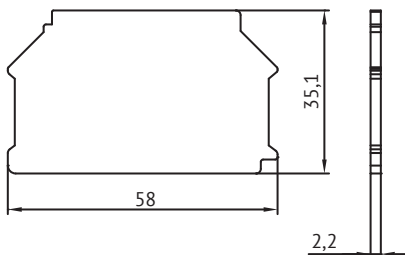
249896 Крышка концевая для клеммы предохранительной OptiClip D-TB-4-NEI-серый
