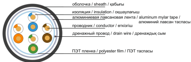
Рисунок 4 – Конструкция кабеля типа F/UTP (количество жил 4x2) / Figure 4 – Cable design of F/UTP type (number of cores 4x2) / Сурет 4 – F/UTP типті кабель дизайны (4x2 талсымдар саны)
