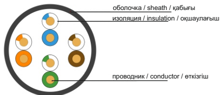
Рисунок 2 – Конструкция кабеля типа U/UTP (количество жил 4x2) / Figure 2 – Cable design of U/UTP type (number of cores 4x2) / Сурет 2 – U/UTP типті кабель дизайны (4x2 талсымдар саны)
