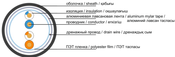
Рисунок 3 – Конструкция кабеля типа F/UTP (количество жил 2x2) / Figure 3 – Cable design of F/UTP type (number of cores 2x2) / Сурет 3 – F/UTP типті кабель дизайны (2x2 талсымдар саны)
