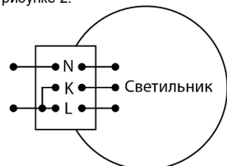
Рис. 2 Схема подключения
