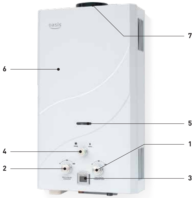
Рис. 1. Аппарат водонагревательный проточный газовый бытовой «OASIS» 1 - ручка водяного регулятора; 2 - ручка газового регулятора; 3 - цифровой индикатор температуры горячей воды; 4 - переключатель зима/лето; 5 - окно смотровое; 6 - облицовка; 7 - патрубок дымоотвода.
