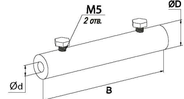
Зажим продольный
