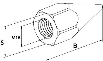
Наконечник заземлителя
