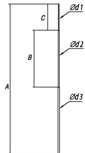
Мачты 8–10 метров
